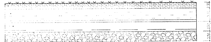
ДЕТАЙЛ 1 ДЕТАЙЛ НА РЕКУЛТИВАЦИОННИ СЛОЕВЕ ВАРИАНТ 1 М 1:50
