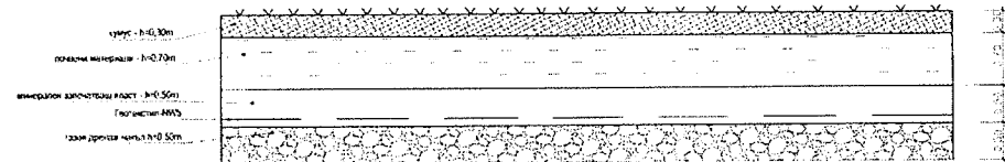
ДЕТАЙЛ 1 ДЕТАЙЛ НА РЕКУЛТИВАЦИОННИ СЛОЕВЕ ВАРИАНТ 2 М 1:50
